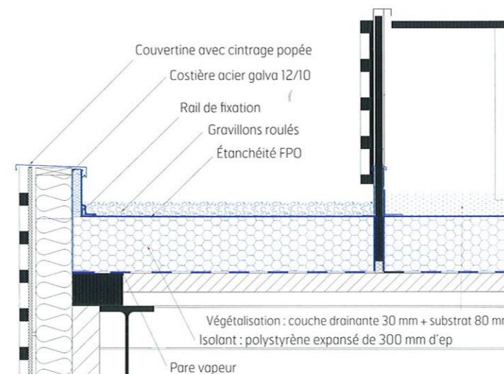
Coupe sur végétalisation
